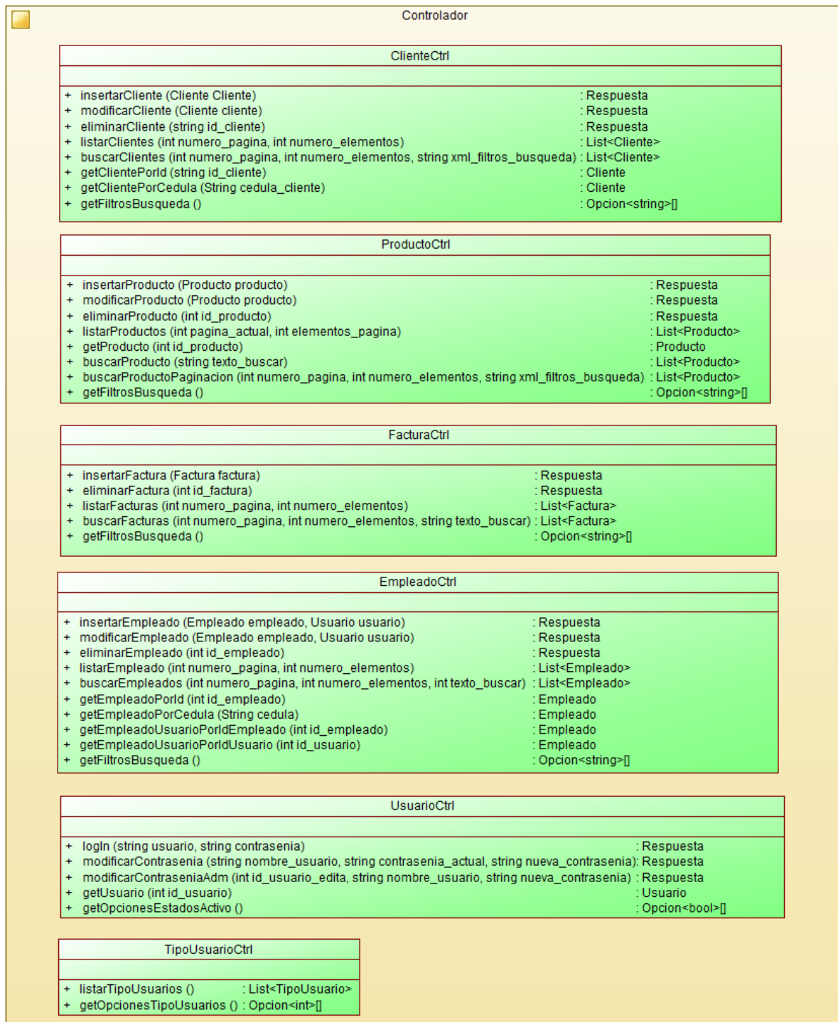
Fig. 29. Diagrama de clases – Paquete de Controladores V1.1
