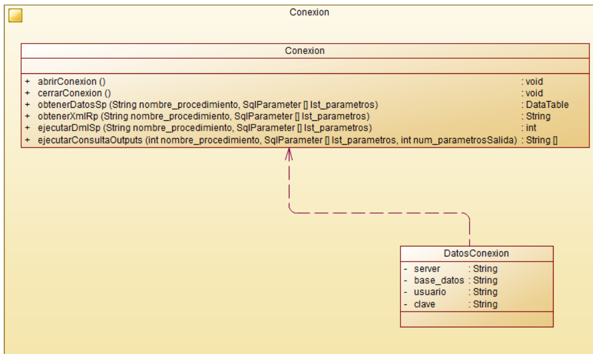
Fig. 28. Diagrama de clases – Paquete de conexión V1.1
